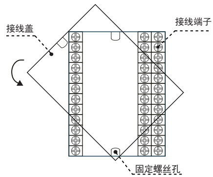
仪表背面图
