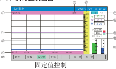
固定值控制
